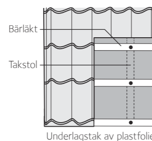
Underlagstak av plastfolie eller board
